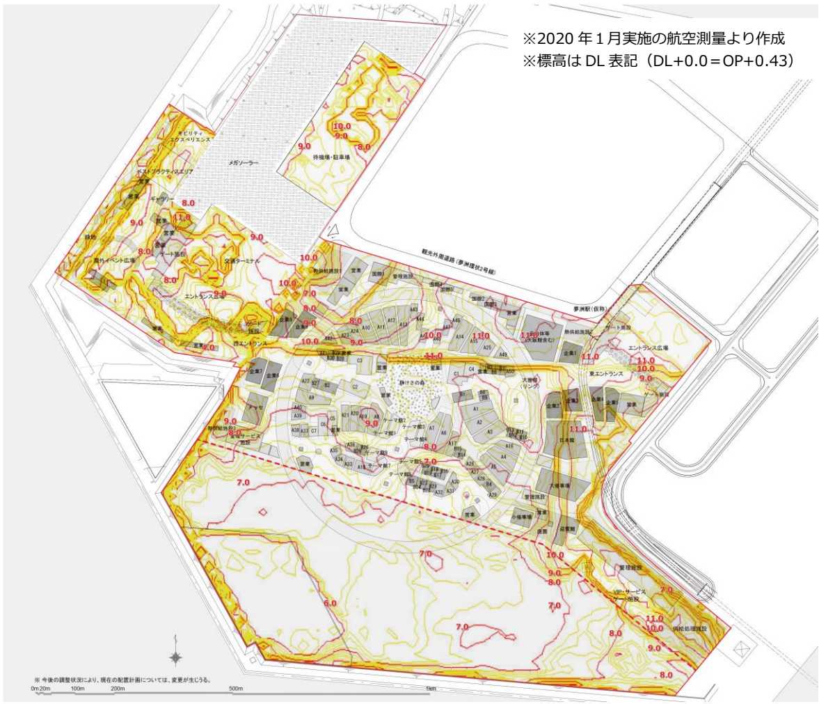
現況地盤高図 (コンター図) 基本計画レイアウト入り
