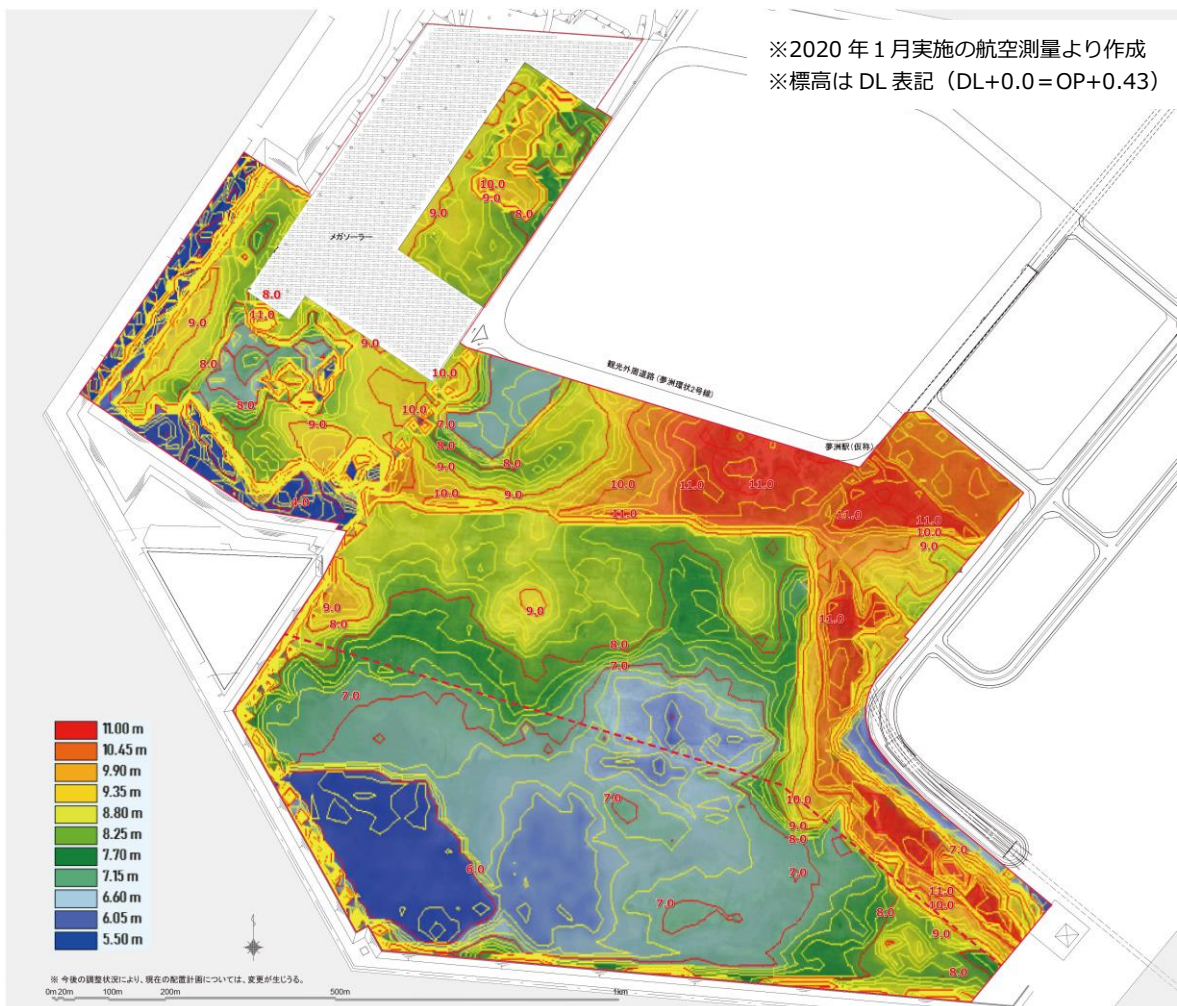
現況地盤高図 (カラーコンター図)
