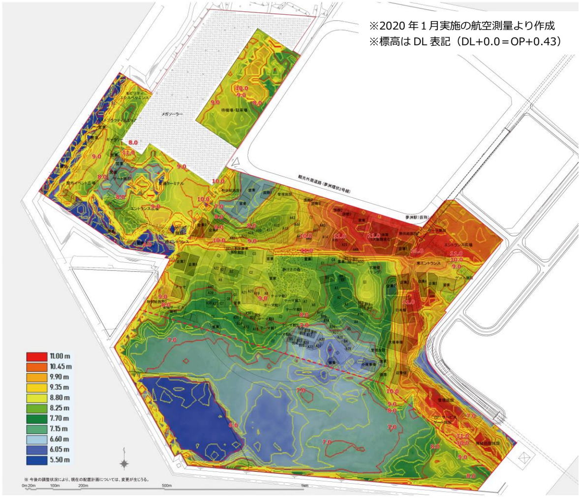
現況地盤高図 (カラーコンター図) 基本計画レイアウト入り
