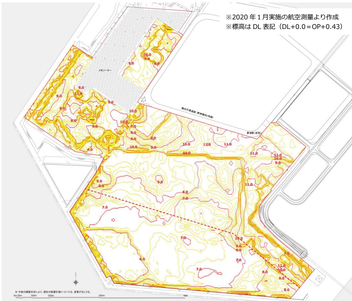
現況地盤高図 (コンター図)
