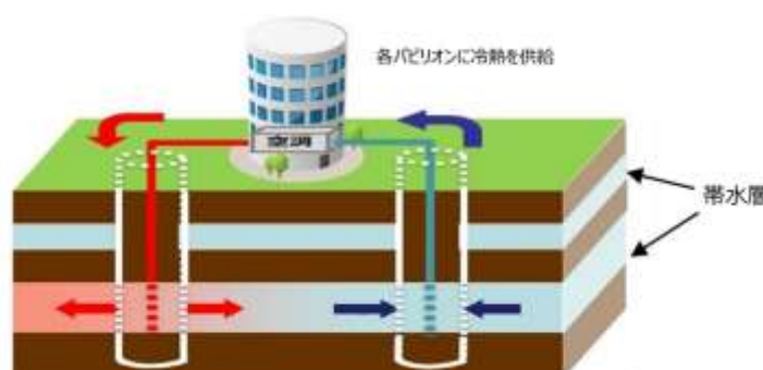
図 3-8 帯水層蓄熱のイメージ (大阪市環境局、在大阪オランダ王国総領事館資料より抜粋)
