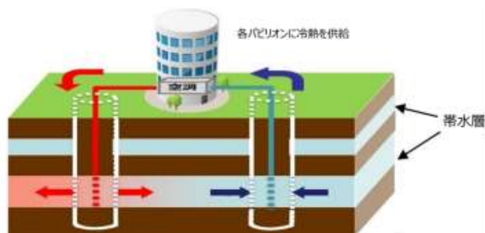
図 3-118 帯水層蓄熱のイメージ (大阪市環境局、在大阪オランダ王国総領事館資料より抜粋)
