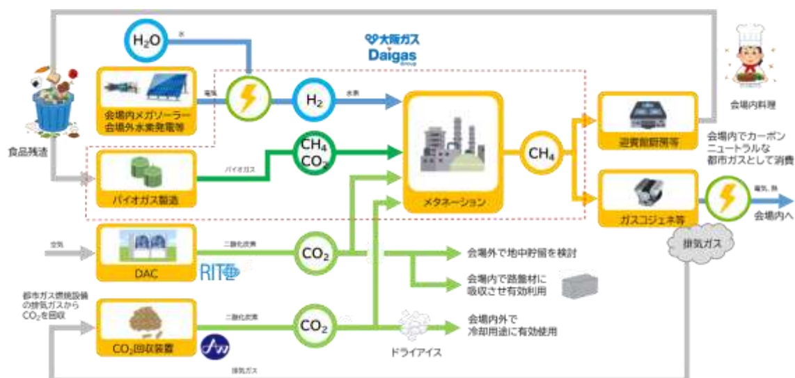
図 3-105 カーボンリサイクルファクトリーの概要
