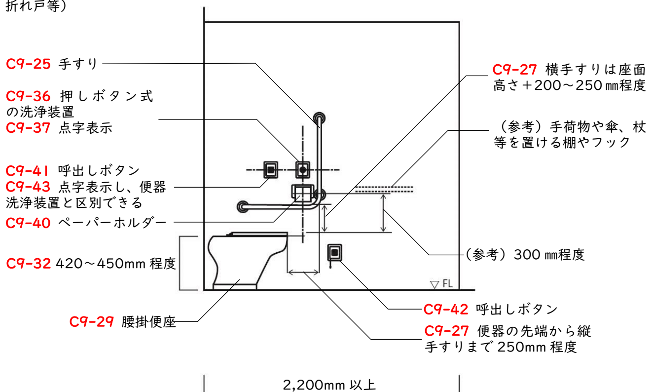
図 3.9.1 車いす使用者用便房の計画例
