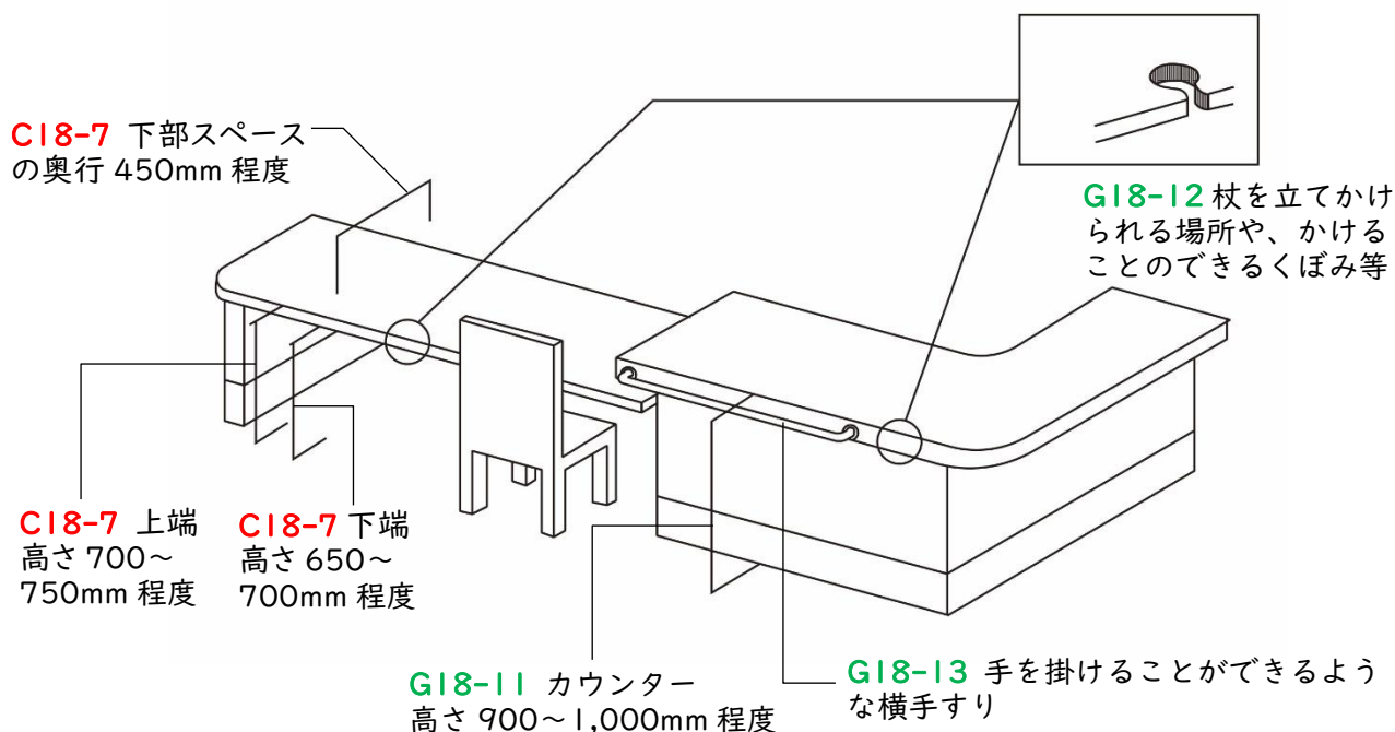
図 3.18.5 カウンターの例
