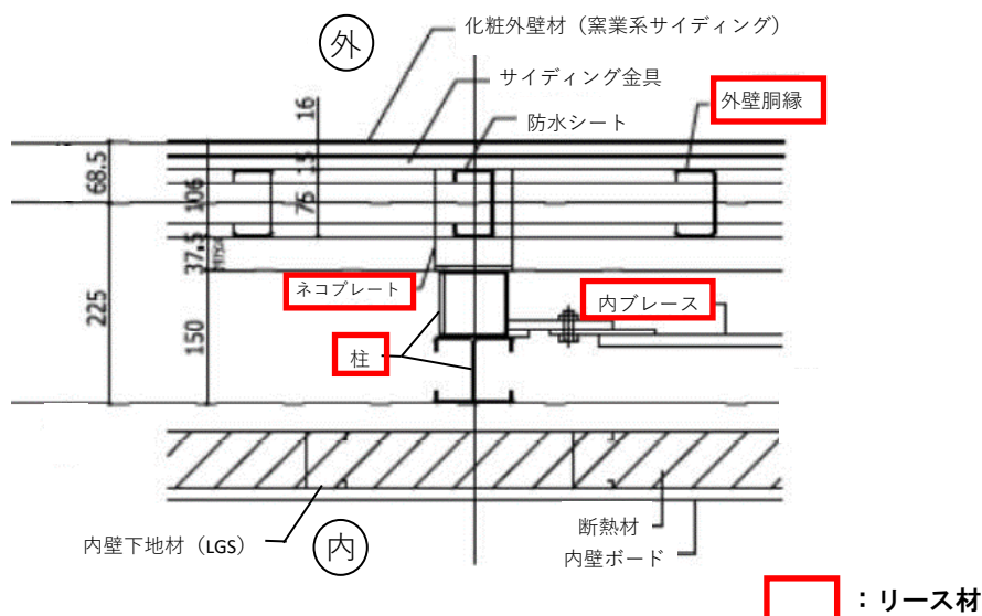
図 2.1 外壁詳細図
