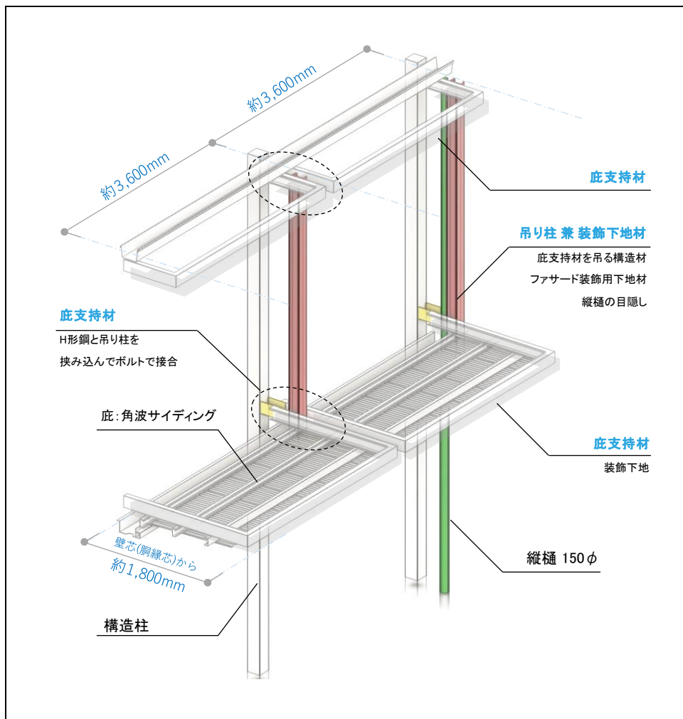
図 2.3 装飾用の下地フレーム（今後変更される可能性があります。）
