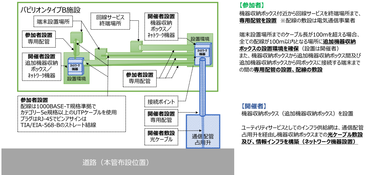
図 4.3 通信インフラの工事区分例
