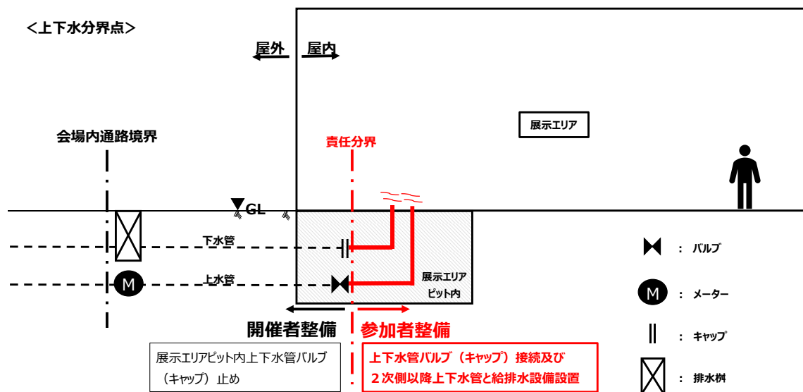
図 4.1 会場内通路境界付近の上下水分界点
