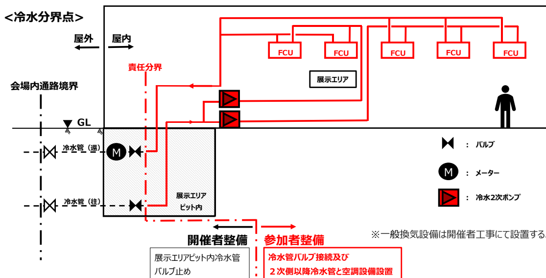
図 4.4 会場内通路境界付近の冷水区分弁
