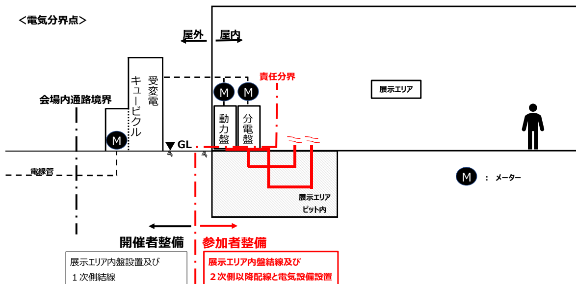
図 4.2 会場内通路境界付近の電気分界点
