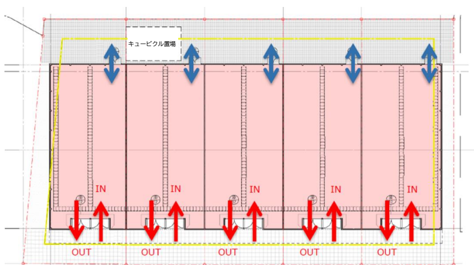
平面計画図
