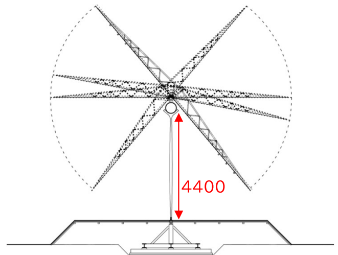
側面図
