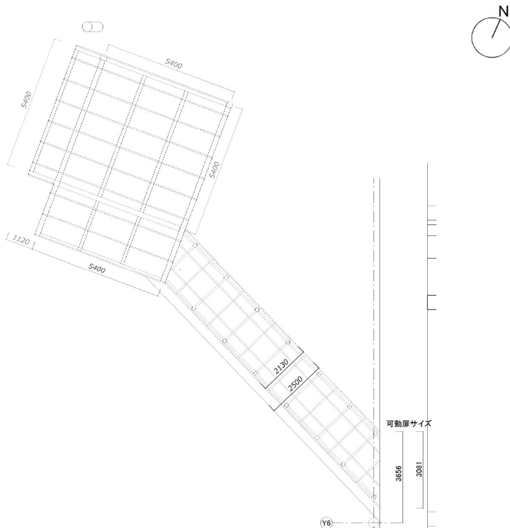
舞台平面図
