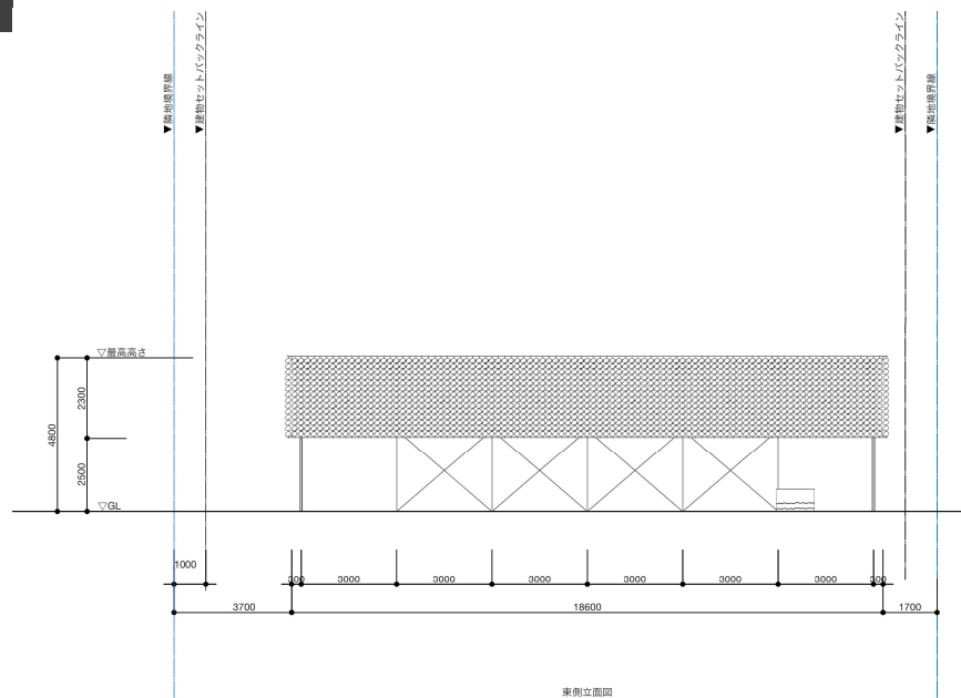
物販棟立面図
