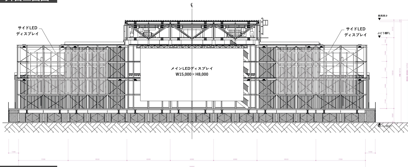
舞台断面図
