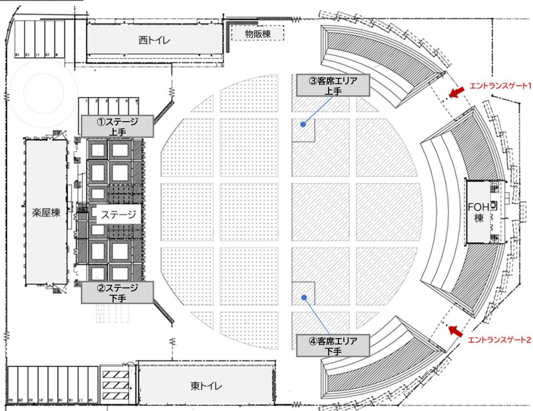
仮設電源配置図
