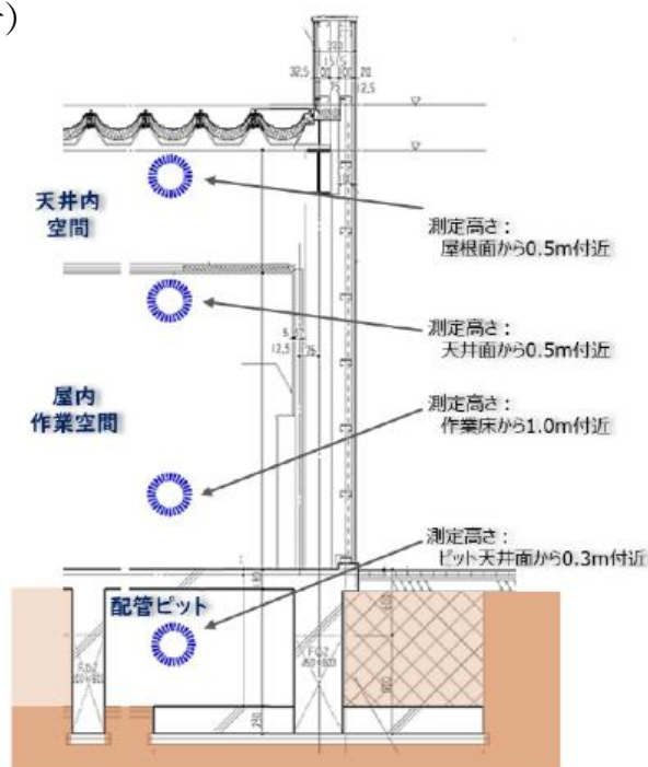
〔図8: 建物の測定箇所のイメージ図〕
