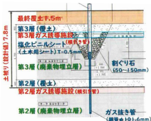
〔図4:ガス抜き管 断面イメージ図 〕
