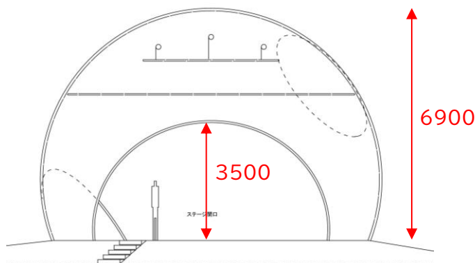
正面図
