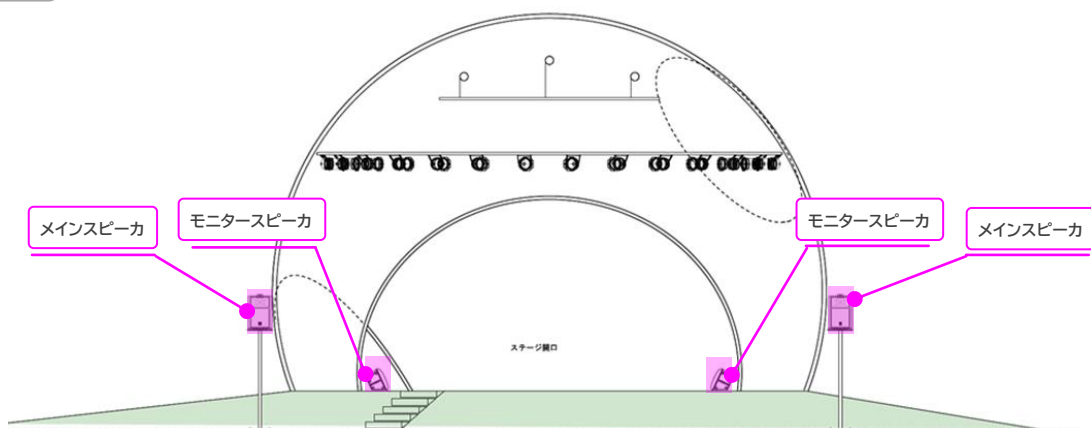
正面図
