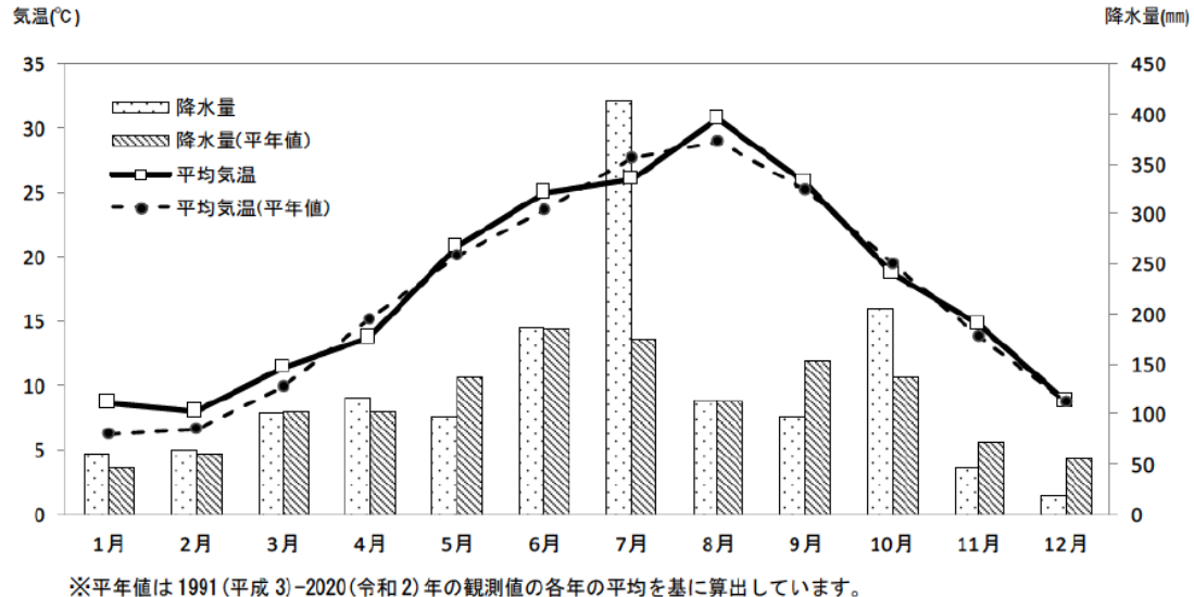
図8 大阪の平均気温、降水量(令和2年・平年) 18
