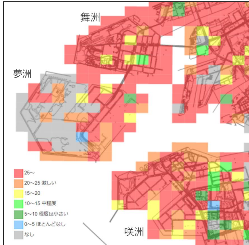
図4 南海トラフ巨大地震による液状化予測図 5
