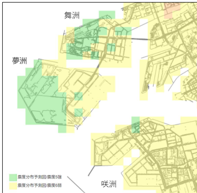
図1 上町断層帯地震における震度分布 2
