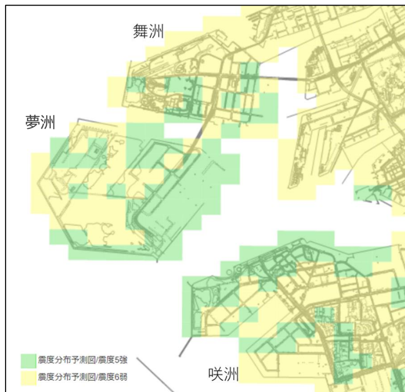
図3 南海トラフ巨大地震における震度分布 4
